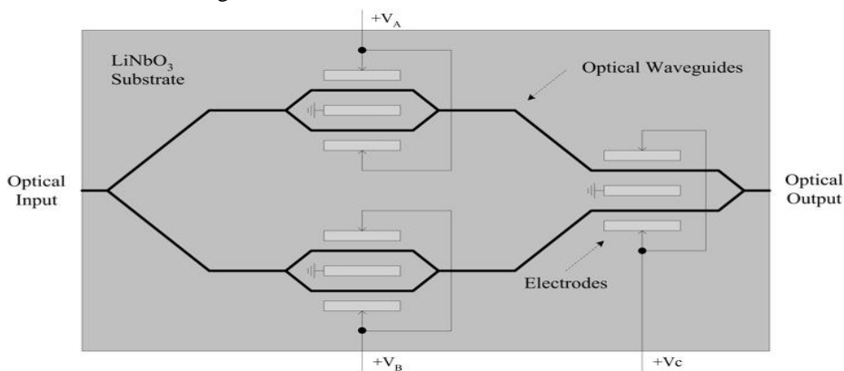
Fig. 3. LiNb MZ modulator
